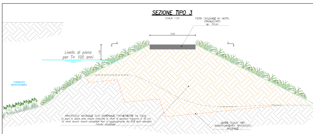
Figura 4. Sezione tipologica di intervento “3”.
