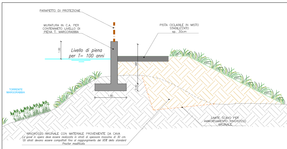
Figura 3. Sezione tipologica di intervento "2".
