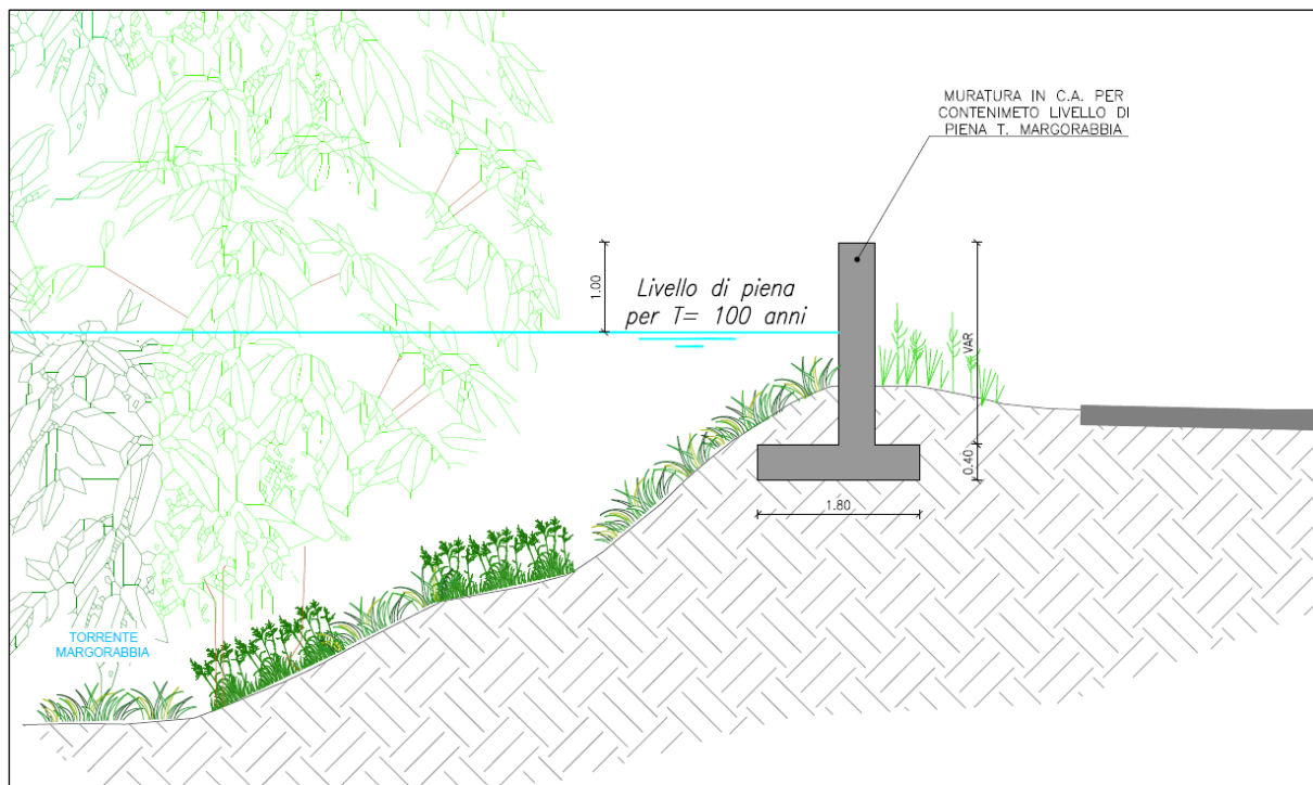
Figura 2. Sezione tipologica di intervento tipo "1"
